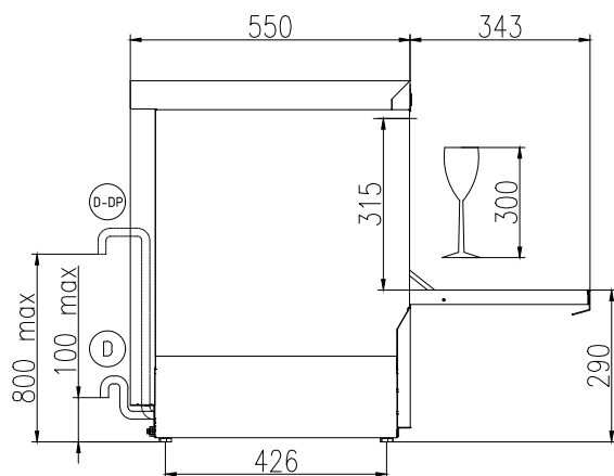
Zij aanzicht
